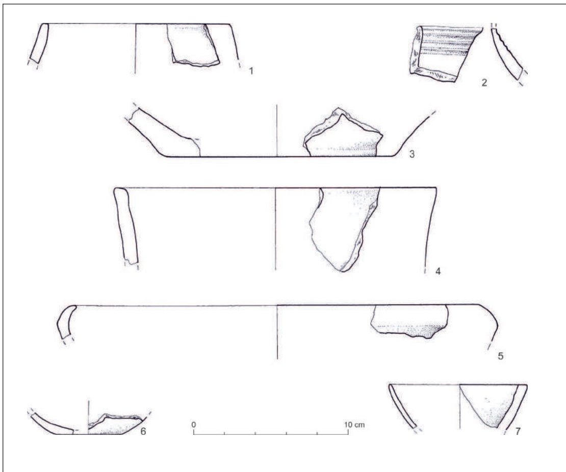
Obr. 4. Kotmanová (Pohanský hrad). Výber keramiky kyjatickej kultúry. Kresba: J. Marettová. Fig. 4. Kotmanová (Pohanský hrad). Selection of the Kyjaticke Culture pottery. Drawing: J. Marettová.
