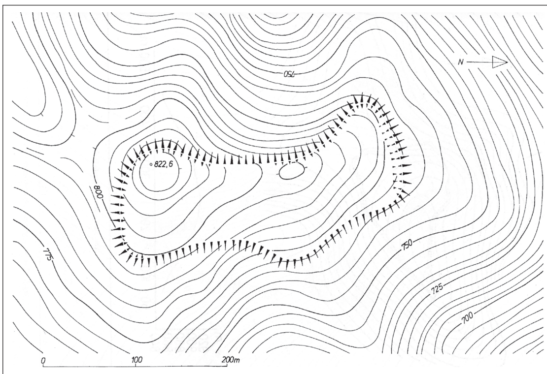
Obr. 5. Plán hradiska kyjatickej kultúry Diósjenő-Pogányvár (podľa Matuz D./Nováki 2002). Fig. 5. Plan of the Kyjaticke Culture hill-fort Diósjenő-Pogányvár (after Matuz D./Nováki 2002).
